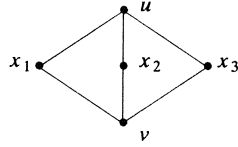
Fig. 4.3A: K_{2,3}
